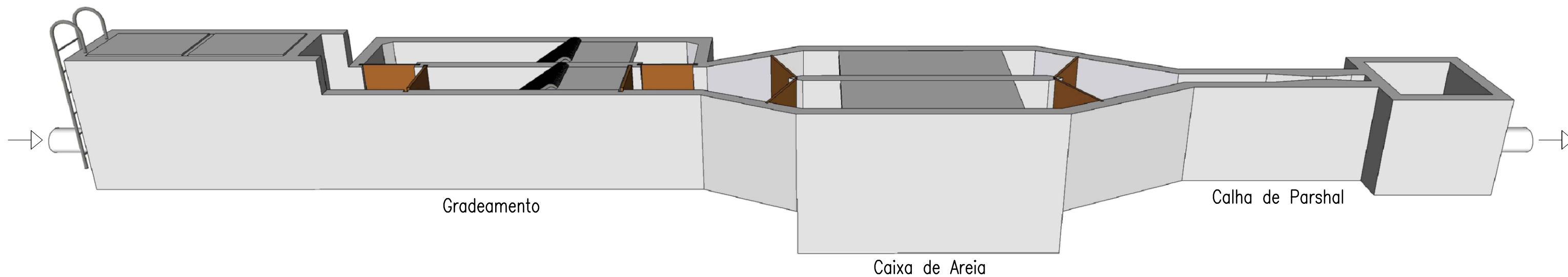
Perspectiva – Gradeamento/Caixa de Areia/Calha de Parshal escala 1/50
