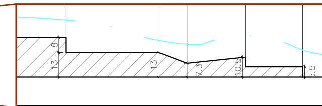
Detalhe – Calha de Parshal escala 1/20
