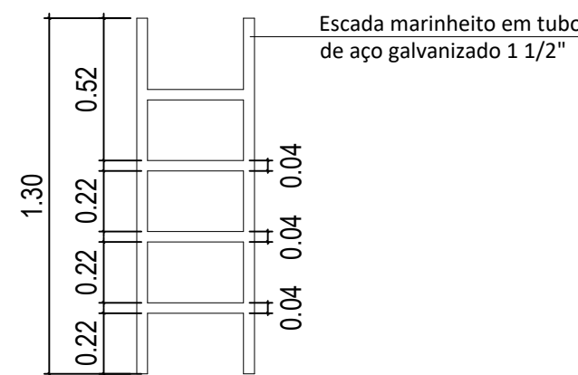
Detalhe – Escada Marinheiro escala 1/25
