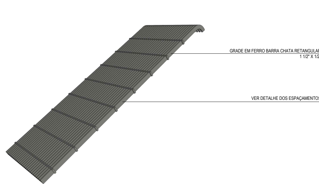
Perspectiva – Gradeamento escala 1/50
