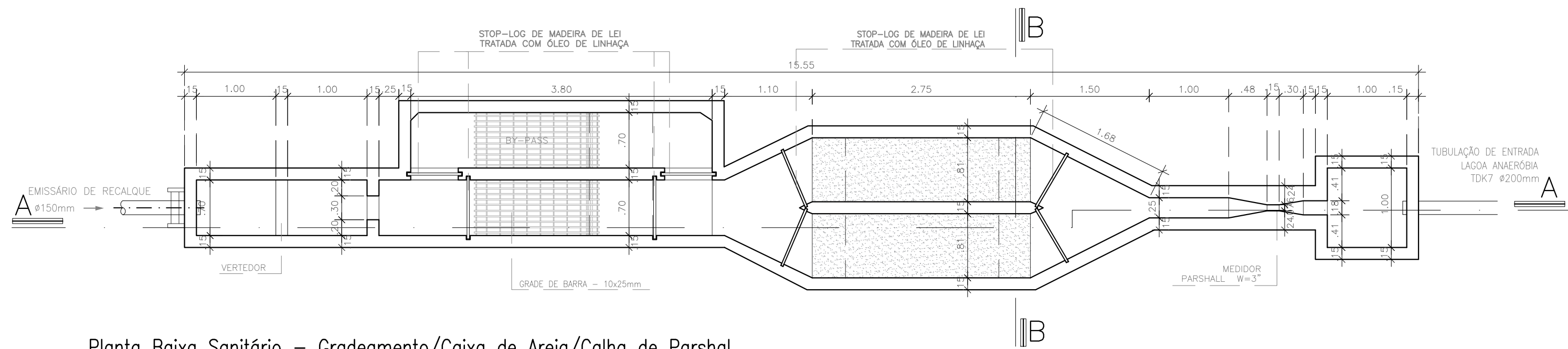
Planta Baixa Sanitário – Gradeamento/Caixa de Areia/Calha de Parshal escala 1/50
