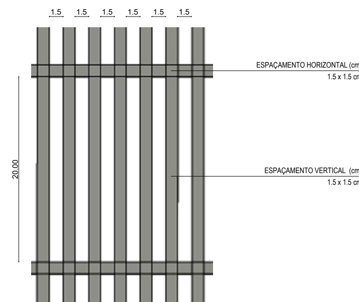
Detalhe – Espaçamento escala 1/25
