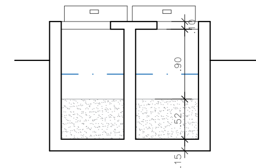
Corte BB – Caixa de Areia escala 1/50
